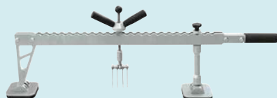
Barre de débosselage double action ref. 053564
