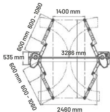
DM4.OEM-EL 4 BRAZOS ARTICULADOS EV 4 ARTICULATED EV ARMS 4 BRAS ARTICULÉS EV
