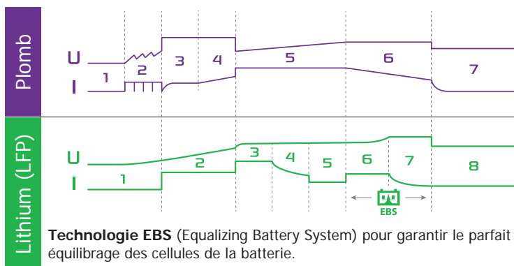
Courbe de charge spécifique en 7 étapes sans surveillance.
